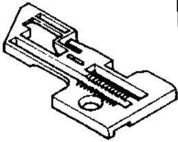
33540 D1 33541 D2 33531 D4
